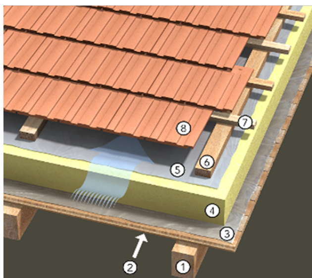
Abbildung 1: Aufbau einer Aufsparrendämmung (Energie Agentur Steiermark)
