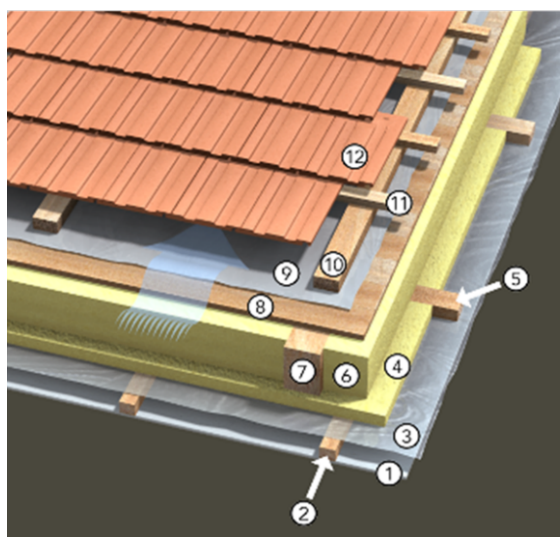
Abbildung 2: Aufbau einer Zwischensparrendämmung (Energie Agentur Steiermark)
